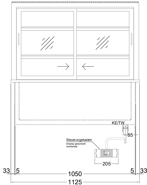
(Bedienseite)
