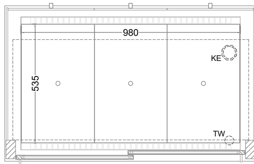
(Grundriss)
