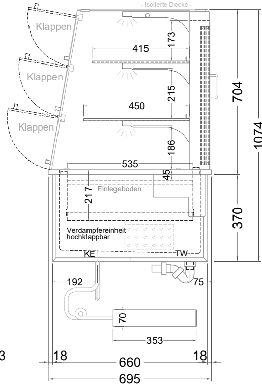
(Seitenansicht)
