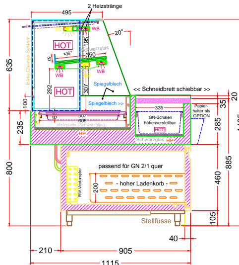
(Schnitt A-A)
