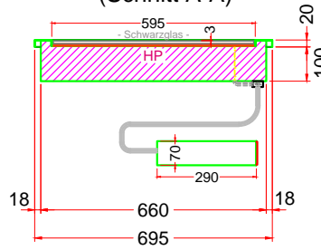
(Schnitt A-A)
