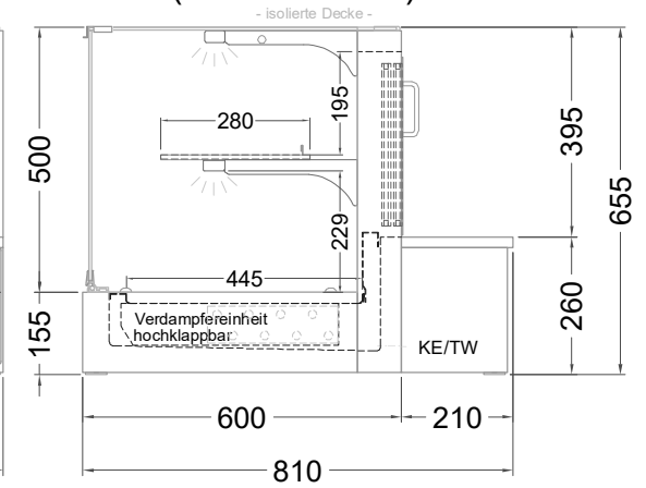
(Seitenansicht)
