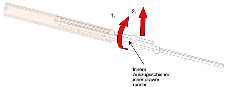
Abbildung 9: Auszugsschiene drehen.
