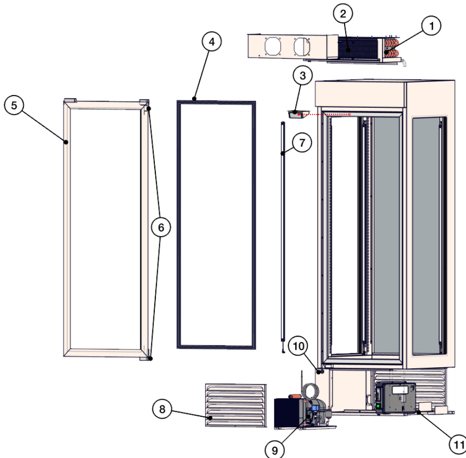
Abbildung 16: Teileübersicht
