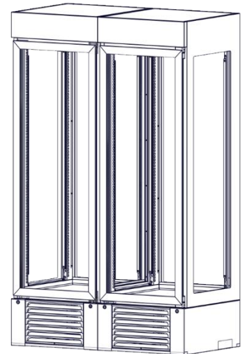
Abbildung 13: Schränke verbinden
