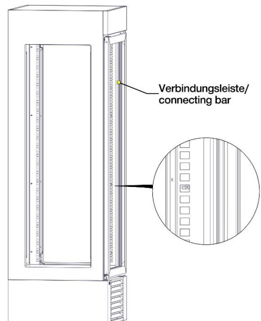
Abbildung 12: Lochleiste_Verbindungsleiste
