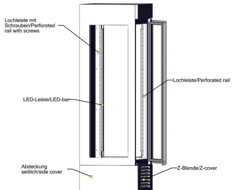
Abbildung 14: Rahmenleisten einsetzen
