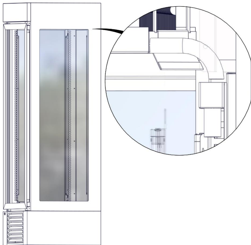
Abbildung 4: Tauwasseranschluss
