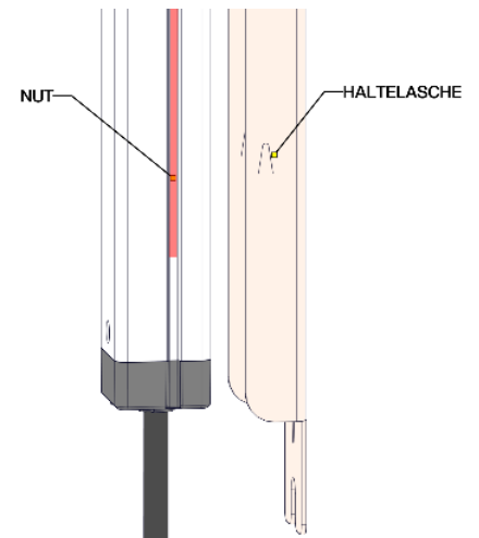
Abbildung 8: LED -Lampe
