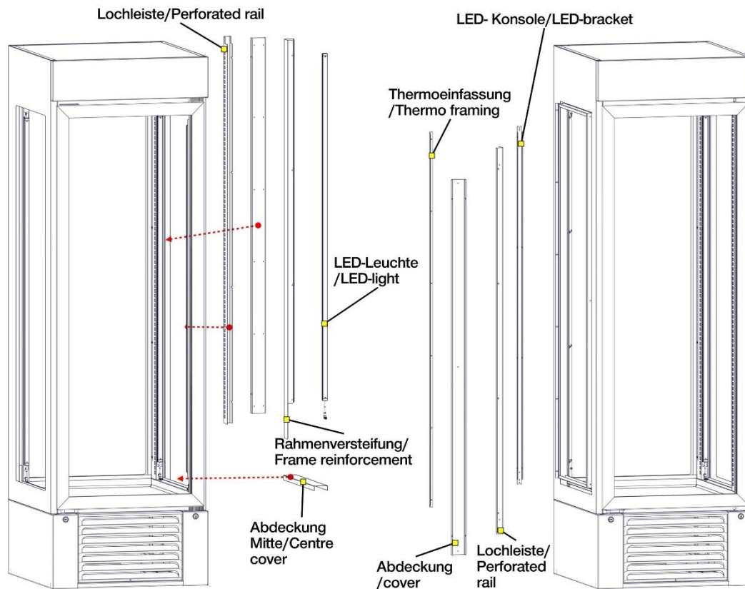
Abbildung 11: Übersicht Teile Zusammenbau
