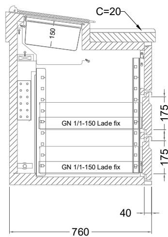
2 Züge 1/3-1/3 mit Blende
