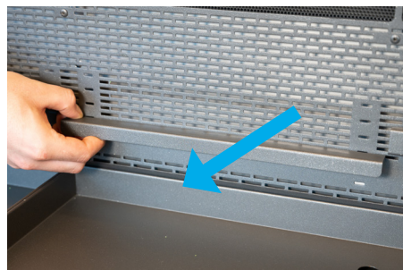
4 Träger befestigen
