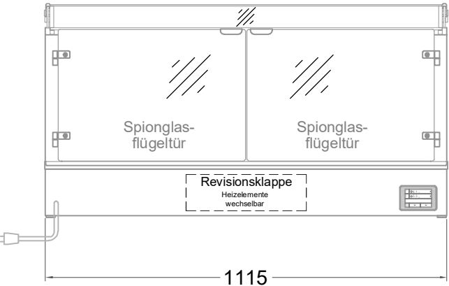
(Bedienseite)
