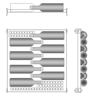
Auflagebord WKS Ausschnitt
