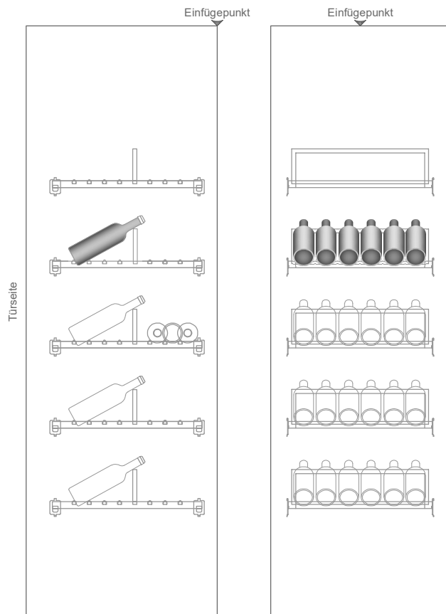
SEITENANSICHT RECHTS
