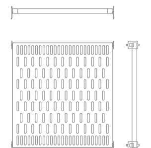
Auflagebord WKS Lochung
