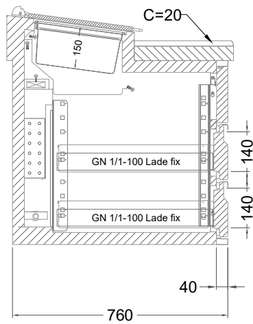
2 Züge 1/3-1/3 mit Blende
