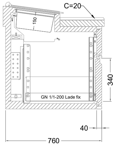
1 Zug mit Blende
