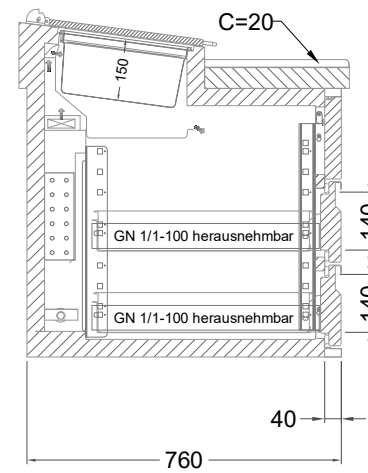
2 Züge 1/3-1/3 mit herausnehmbaren Ladeneinsätzen mit Blende
