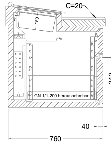
1 Zug mit herausnehmbarem Ladeneinsatz mit Blende
