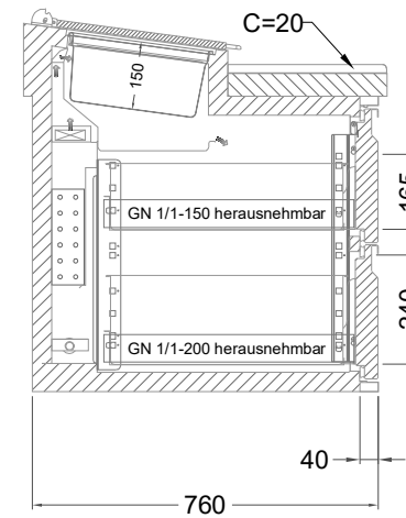
2 Züge 1/2-1/2 mit herausnehmbaren Ladeneinsätzen
