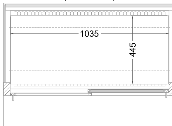
(Grundriss)
