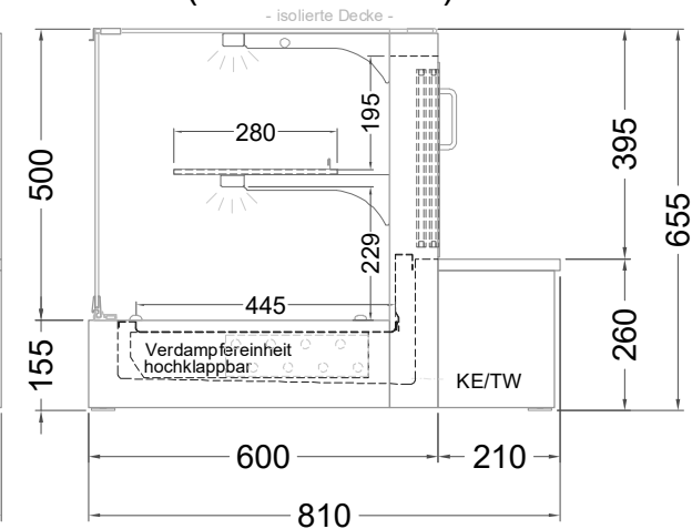
(Seitenansicht)
