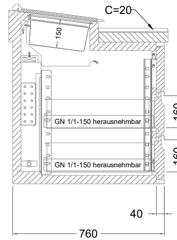
2 Züge 1/3-1/3 mit herausnehmbaren Ladeneinsätzen mit Blende
