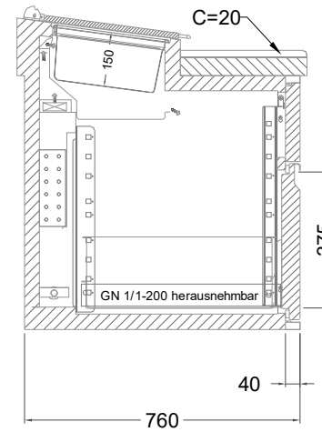
1 Zug mit herausnehmbarem Ladeneinsatz mit Blende
