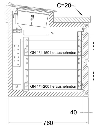
2 Züge 1/2-1/2 mit herausnehmbaren Ladeneinsätzen
