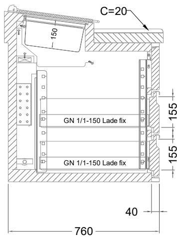
2 Züge 1/3-1/3 mit Blende
