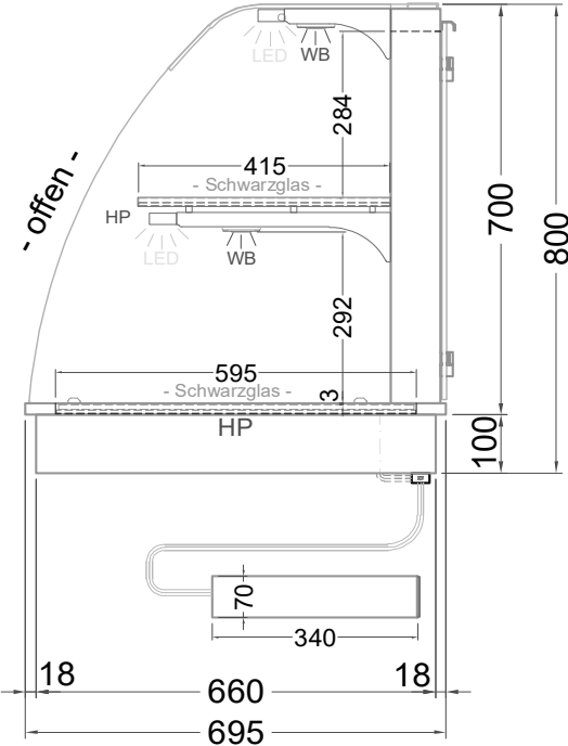
(Seitenansicht)
