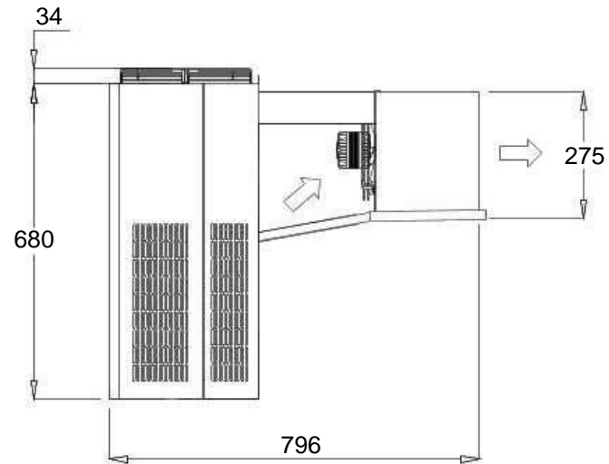
Seitenansicht
