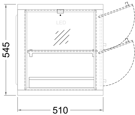
(Seitenansicht)
