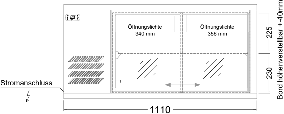
(Bedienseite)
