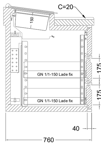
2 Züge 1/3-1/3 mit Blende
