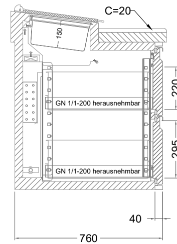
2 Züge 1/2-1/2 mit herausnehmbaren Ladeneinsätzen
