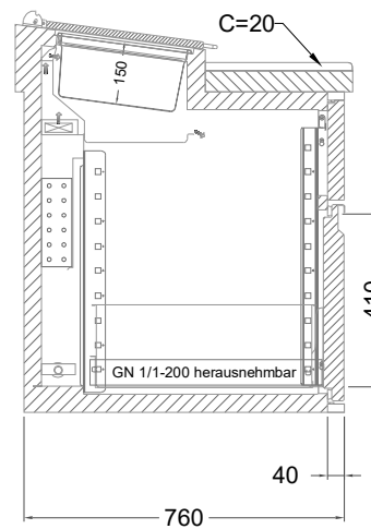
1 Zug mit herausnehmbarem Ladeneinsatz mit Blende
