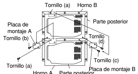
Figura A. Cómo instalar dos hornos
