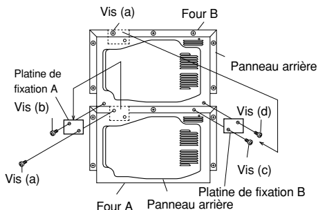
Figure A: Installation de deux fours
