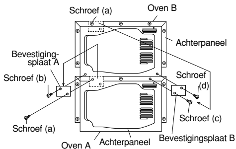
Afbeelding A: Installeren van twee ovens.
