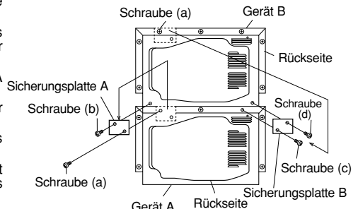
Abb. A: Verschrauben von zwei Mikrowellengeräten
