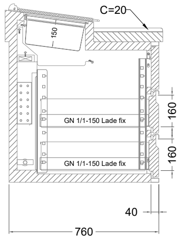
2 Züge 1/3-1/3 mit Blende
