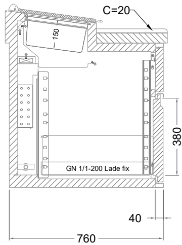
1 Zug mit Blende
