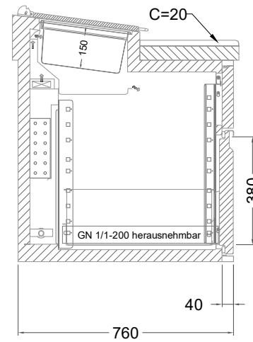
1 Zug mit herausnehmbarem Ladeneinsatz mit Blende
