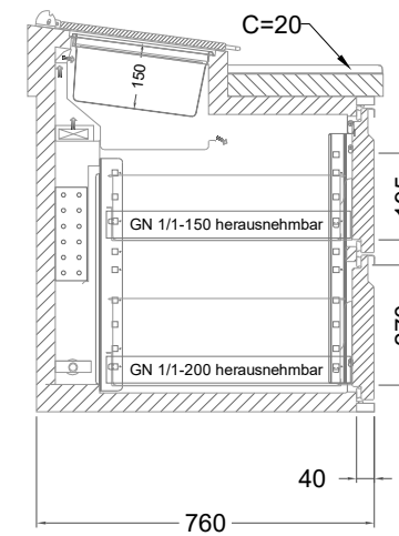
2 Züge 1/2-1/2 mit herausnehmbaren Ladeneinsätzen
