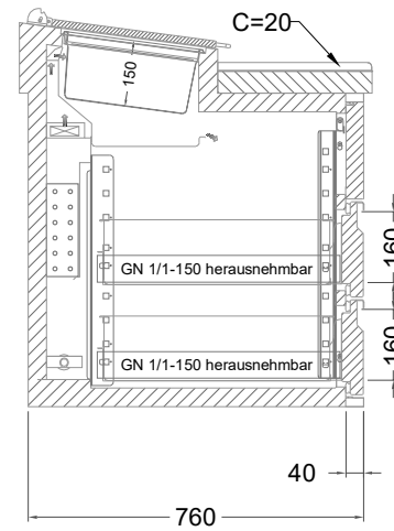
2 Züge 1/3-1/3 mit herausnehmbaren Ladeneinsätzen mit Blende
