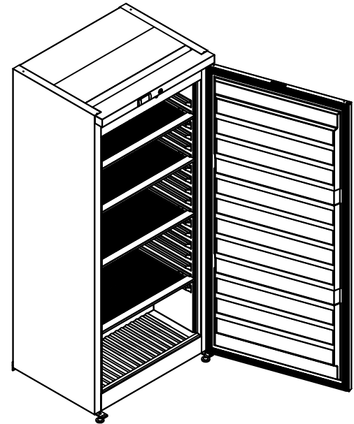
Masszeichnung Backwarentiefkühlschrank BKT 460 [Art. 45111460]
